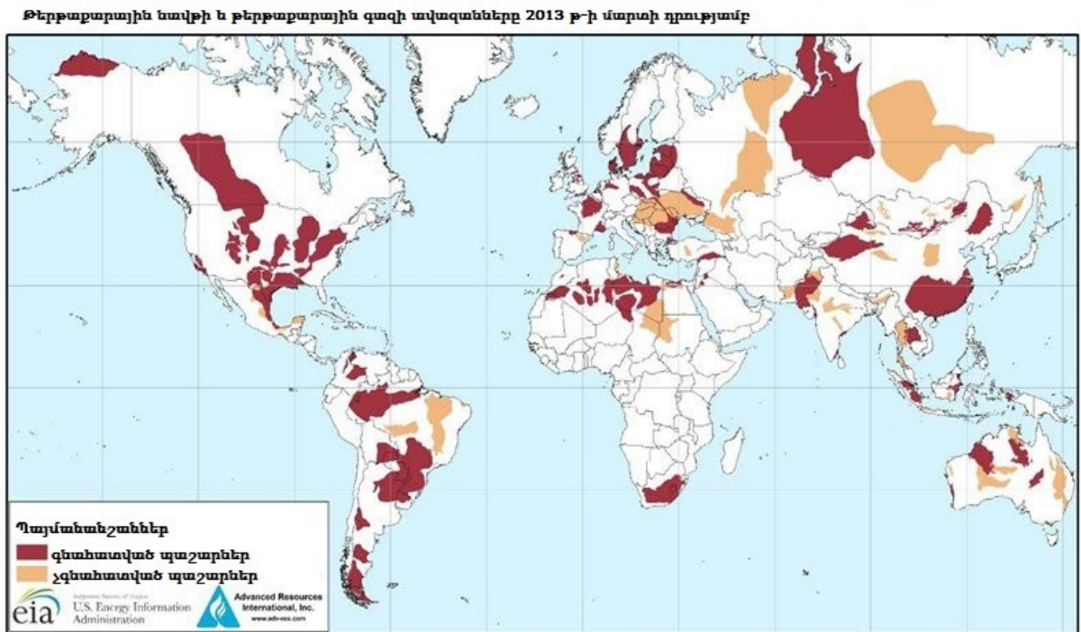
Նկար 1: Թերթաքարային նավթի և թերթաքարային գազի տարածման հիմնական ավազանները
