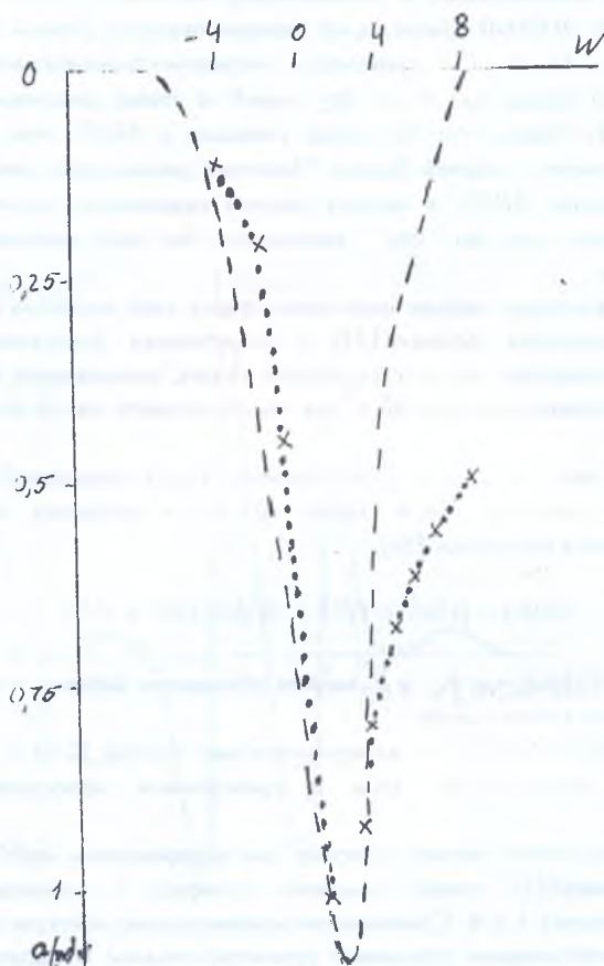
Рис.3. Количественное сравнение экспериментального (пунктирная) и расчетного (точки) контуров линий не прямых экситонных состояний селенида кадмия при 77К.
