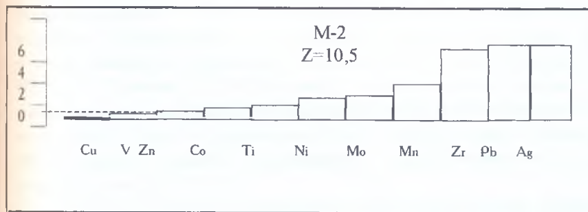
Рис. 2. Гистограммы распределения элементов в почвах Дрмбонского (Д) и Мехманинского (М) участков в единицах кларка почв (Д-1 и М-1) и местного фона (Д-2 и М-2)
